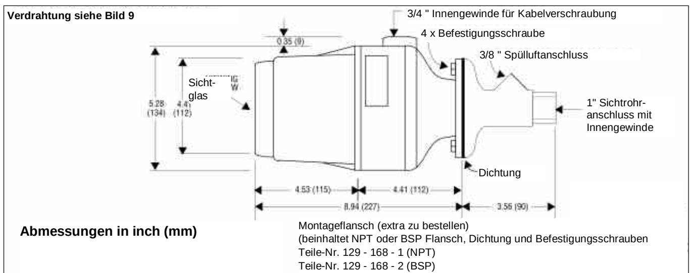
Bild 2: Phoenix Flammenwächter in CENELEC EE x d - Gehäuse
