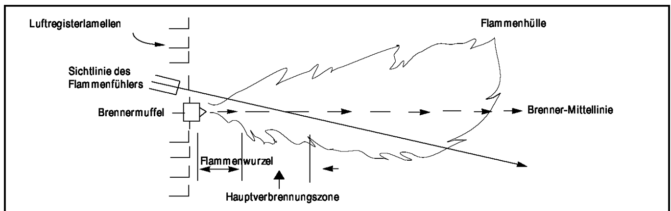
Bild 3: Sichtlinie des Flammenwächters für einen Einzelbrenner
