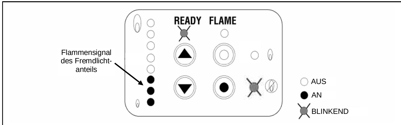
Bild 16: Fremdlichtanteil lernen (Optional)
