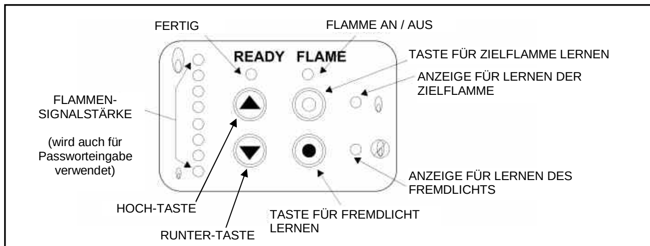
Bild 10: Bedientasten und Funktion der LED
