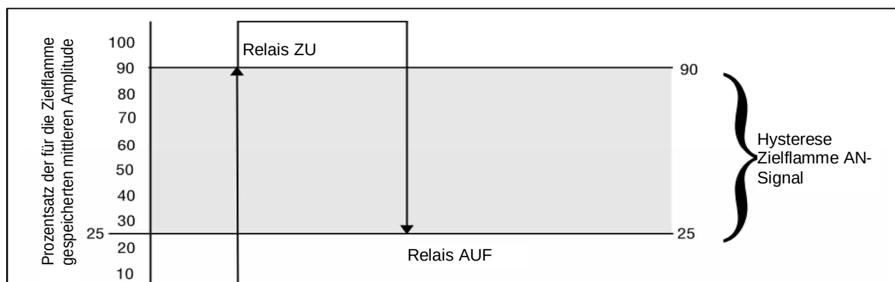
Bild 15: Beispiel für Flammenerkennungsschwellenwerte (nach Durchführung Zielflamme lernen)
