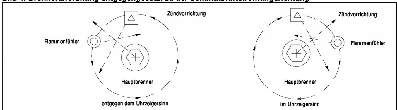
Bild 4: Brenneranordnung entgegengesetzt zu der Sekundärluftströmungsrichtung
