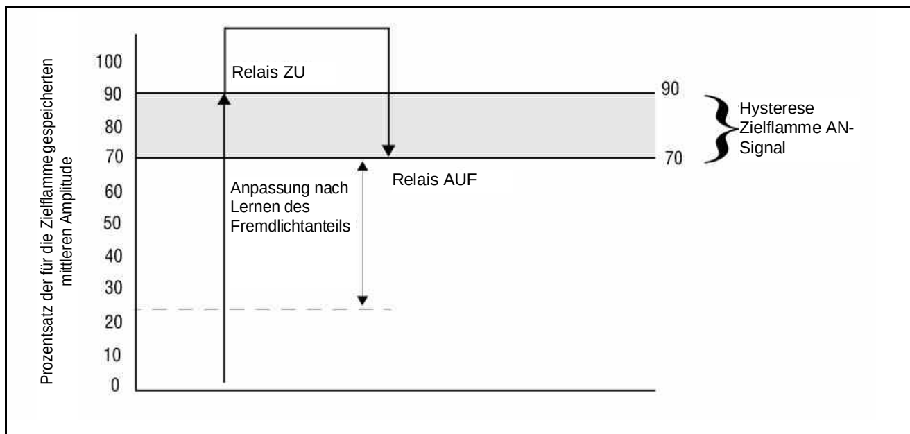
Bild 17: Beispiel für Flammenerkennungsschwellenwerte (Angepasst nach Lernen des Fremdlichtanteils)
