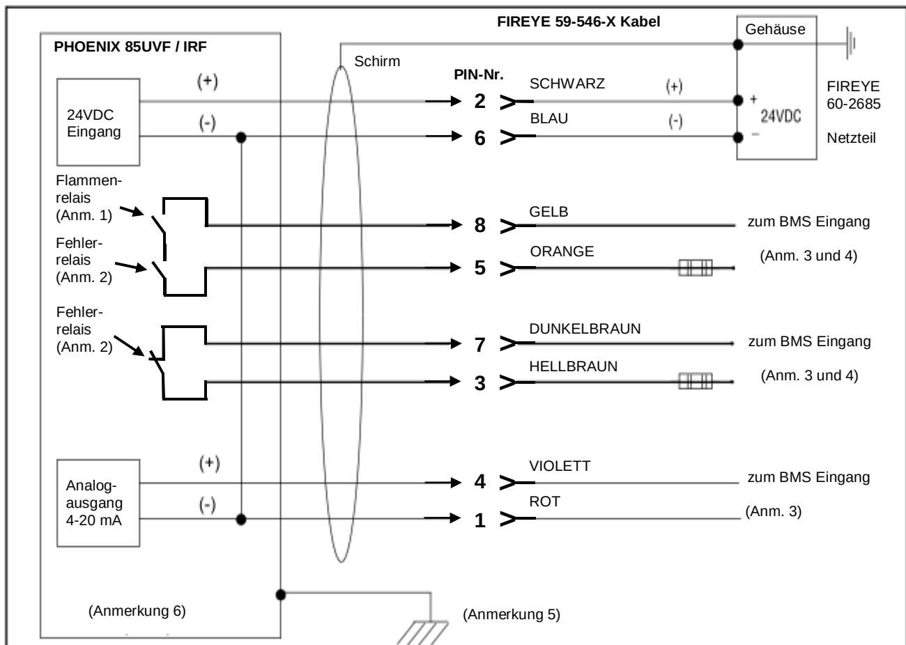
Bild 7: Anschlussplan
