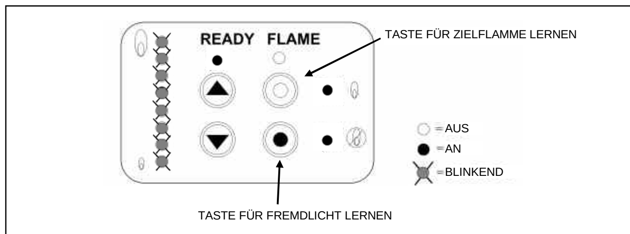
Bild 18: Rücksetzen des Flammenwächters auf herstellerseitigen Auslieferungszustand
