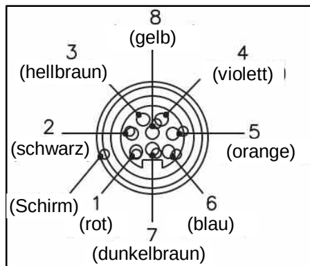
Bild 8: 59-546-X, Pinbelegung der Buchse am Ende des 8adrigen Kabels
