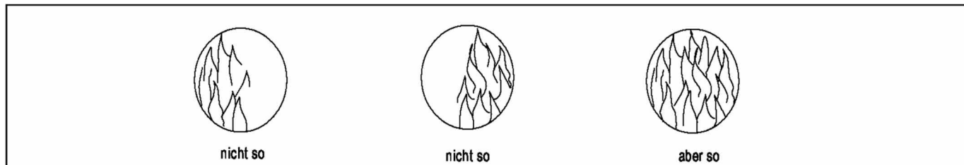
Bild 5: Die Flamme muss die Schauöffnung vollständig ausfüllen
