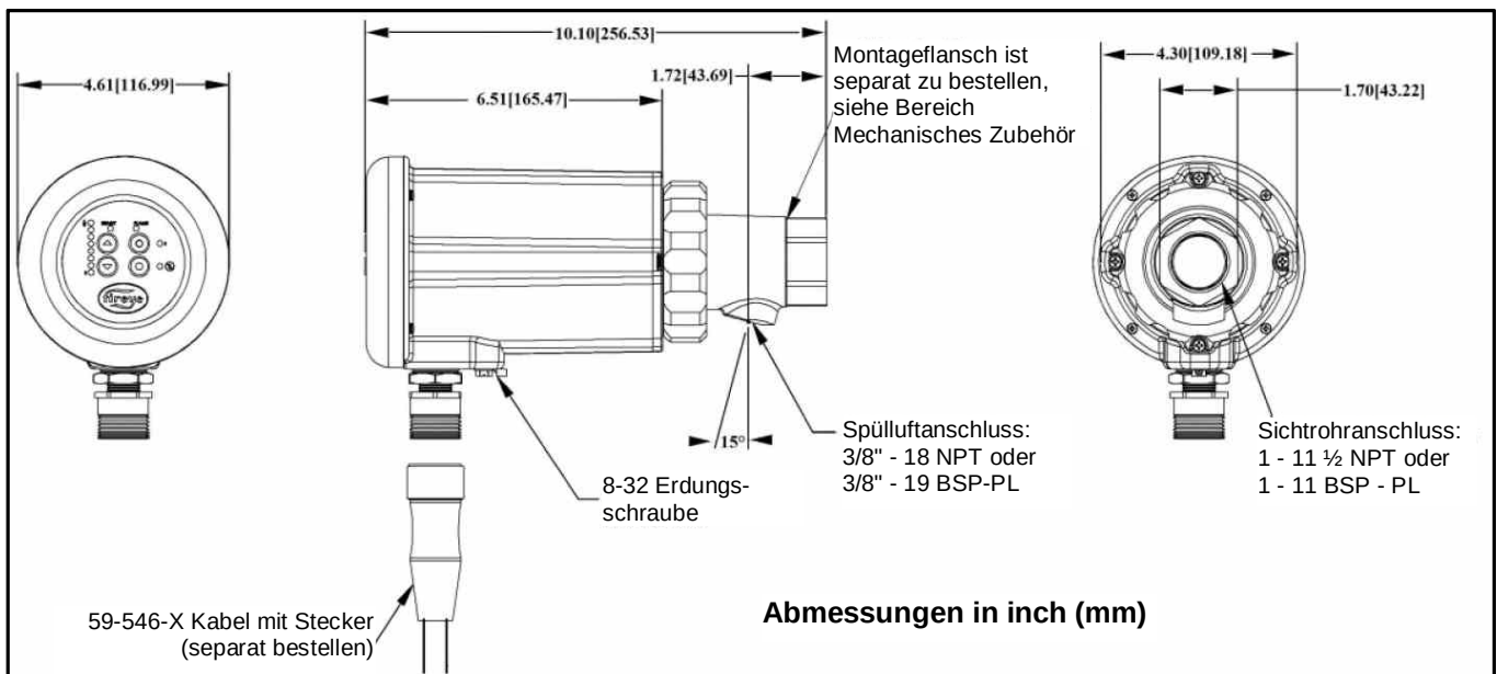
Bild 2: Phoenix Flammenwächter in CENELEC EE x d - Gehäuse
