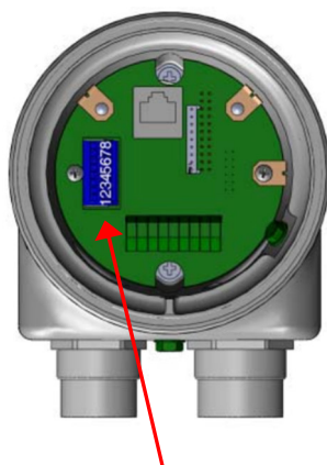
8 poliger Klemmenblock
