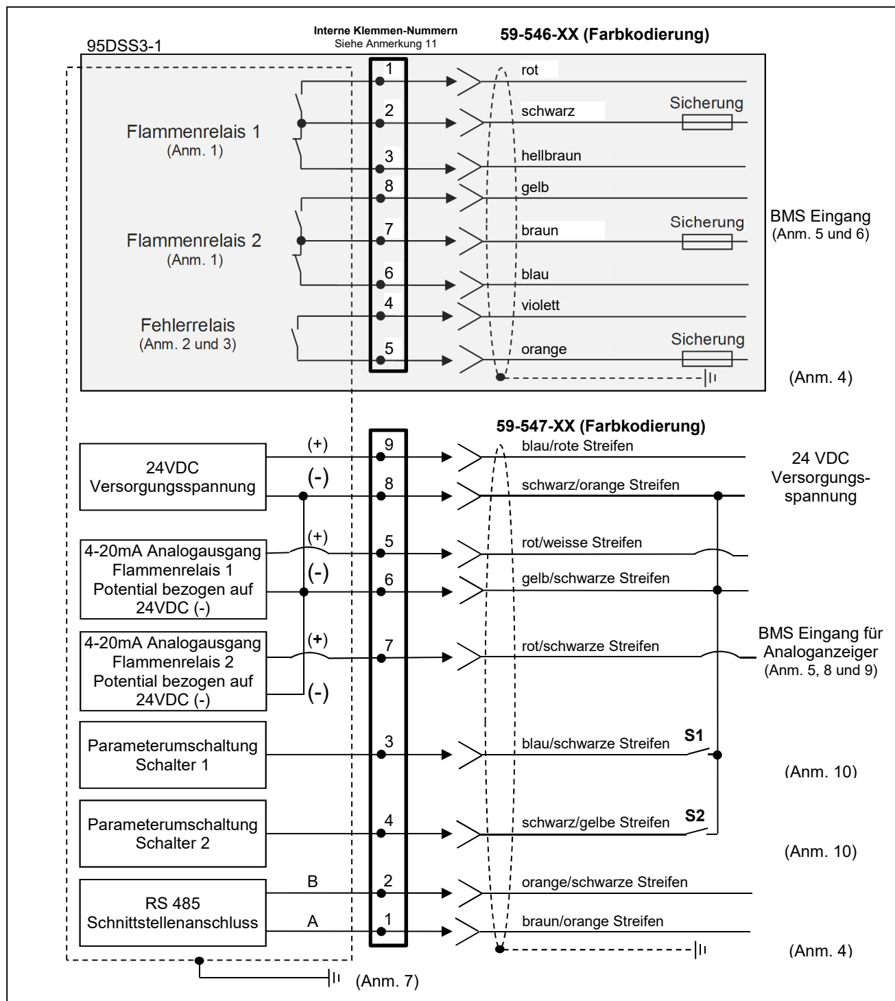
Bild 13 Elektrischer Anschluss 95DSS3-1
