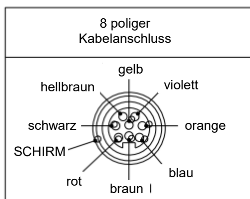
Kabelanschluss 59-546-xx
