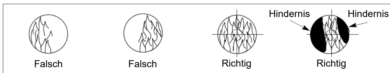
Bild 6 Die Flamme muss die Schauöffnung vollständig ausfüllen
