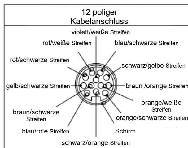
Kabelanschluss 59-547-xx
