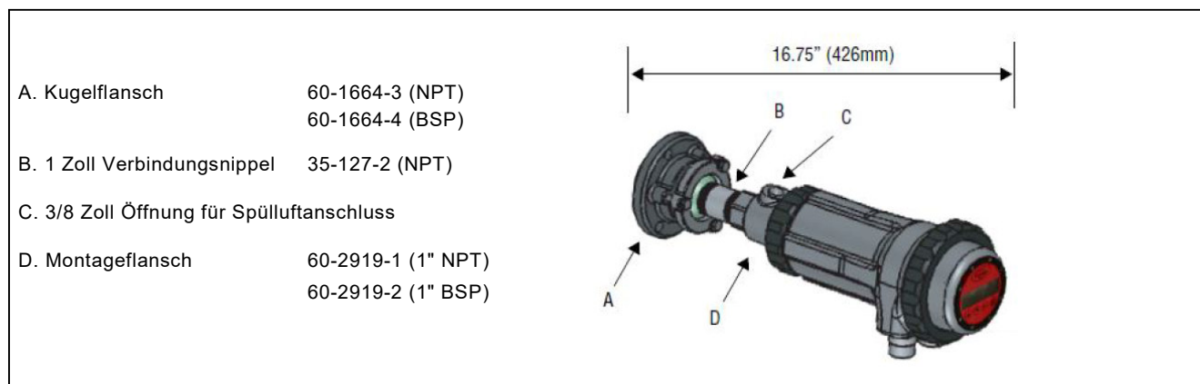
Bild 9 Standardmontage des InSight II
