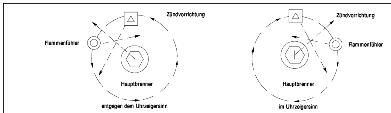
Bild 5 Flammenwächteranbau im Verhältnis zur Sekundärluftströmungsrichtung
