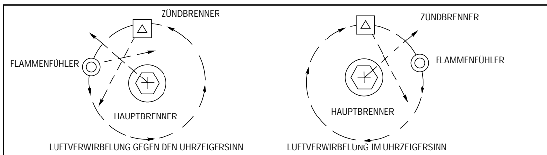
ABBILDUNG 3: POSITIONIERUNG DES FLAMMPFUHlers IN ABHÄNGIGKEIT VON DER SEKUNDÄREN LUFTVERWIRBELUNG
