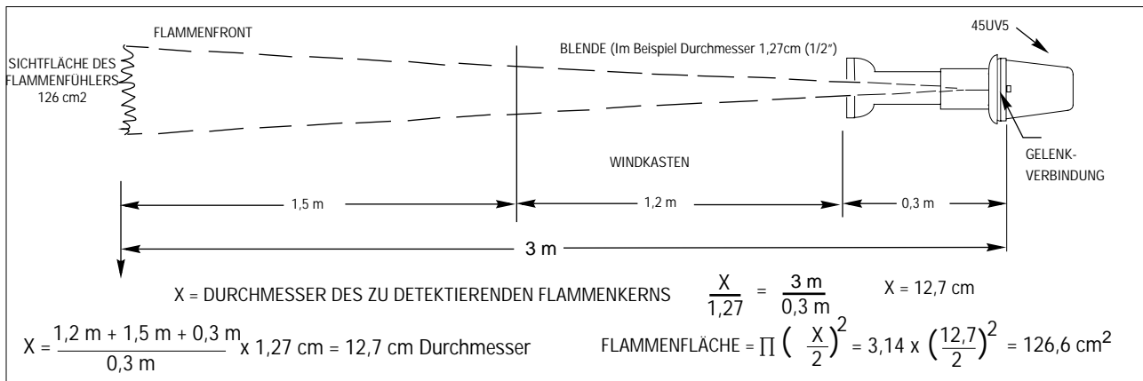
ABBILDUNG 10: FLAMMENFÜHLER MIT BLENDE
