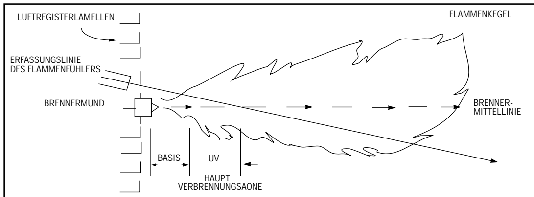
ABBILDUNG 3: POSITIONIERUNG DES FLAMMPFUHlers IN ABHÄNGIGKEIT VON DER SEKUNDÄREN LUFTVERWIRBELUNG
