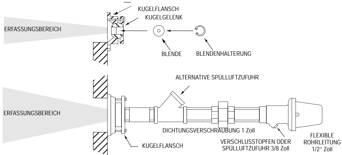
ABBILDUNG 9: BLENDENANORDNUNG
