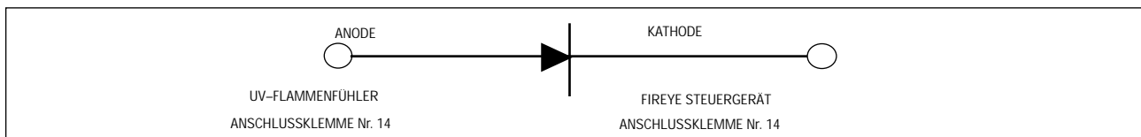
ABBILDUNG 15: SPERRDIODEN-ANSCHLÜSSE
