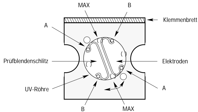
ABBILDUNG 5: POSITION DER UV-RÖHRE
