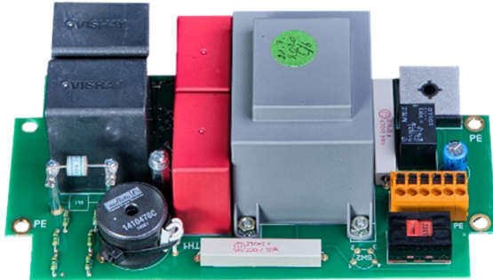
Bild 11: ZSH-GDT: Gasentladediode
