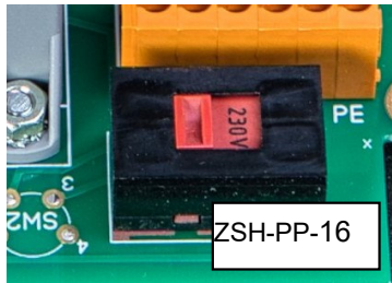
Bild 5: Rastschalter für Umschaltung der Versorgungsspannung
